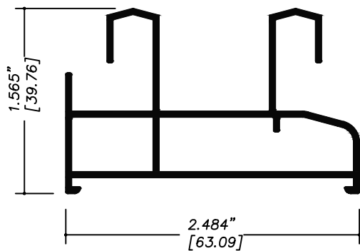
PP4004 RIEL DOBLE
