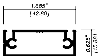
11411 MARCO
