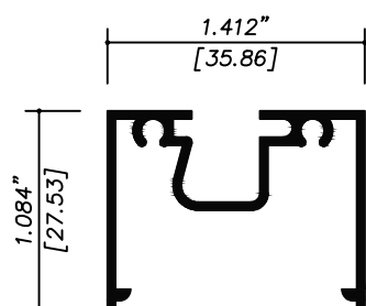
9073 BOLSA
