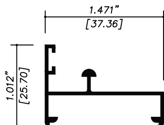
11068 RIEL
