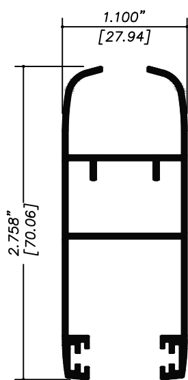
PP4001 HOJA VIDRIO SENCILLO
