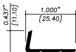
014 RIBETE
