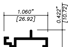
9966 ADAPTADOR MOSQ.
