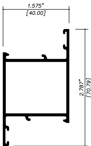
1406 HOJA LISA PUERTA
