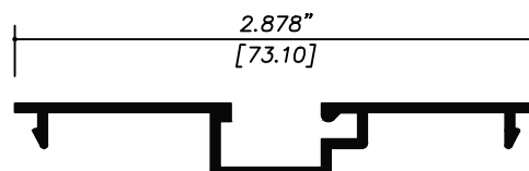
10237 TAPA JAMBA DE 3"
