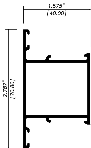
1405 PILASTRA LISA PUERTA
