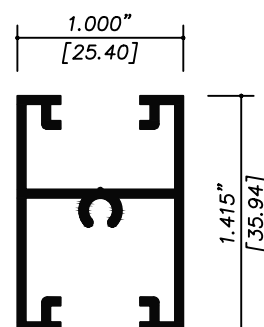
9082 INTERMEDIO
