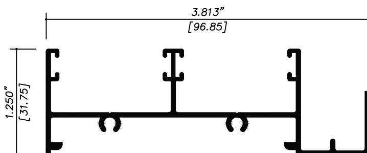
7862 JAMBA CON MOSQ.
