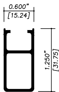
8320 CERCO VENTANA
