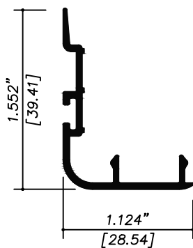
PP4003 TRASLAPE
