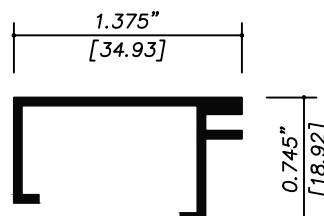
8939 JUNQUILLO
