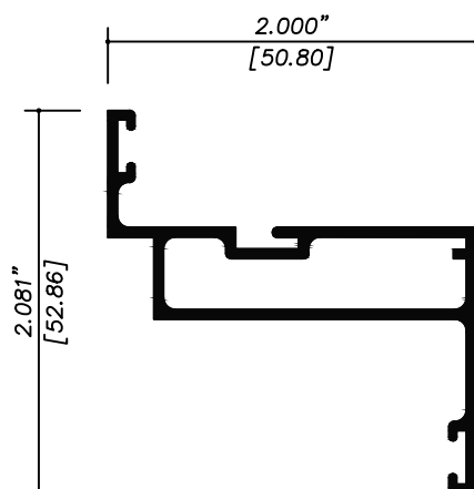
8937 CONTRA MARCO
