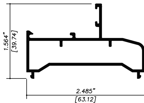
PP4008 FIJO DOBLE
