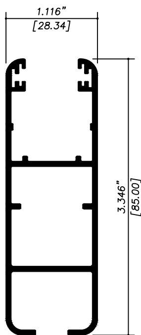
PP42316 HOJA PUERTA
