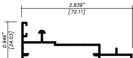
8370 RIEL CON MOSQUITERO
