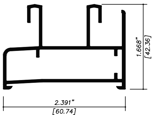
ES01 RIEL DOBLE
