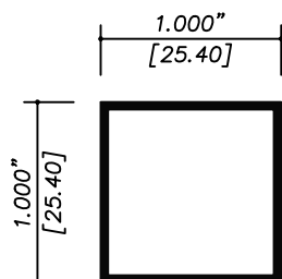
2362 CUADRADO DE 1.00"
