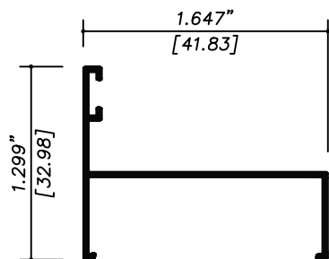
5046 BATIENTE ALTA
