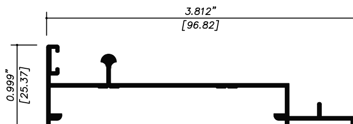
9272 RIEL CON MOSQ. DE 3"
