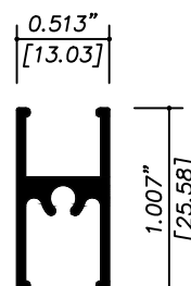
11203 INTERMEDIO CUADRICULA
