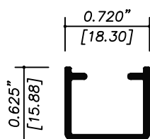
7525 CERCO FIJO ECO.
