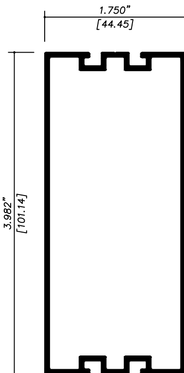
32216 INTERMEDIO PUERTA
