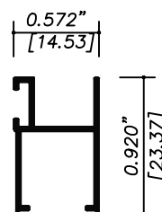
5281 CERCO TRASLAPE
