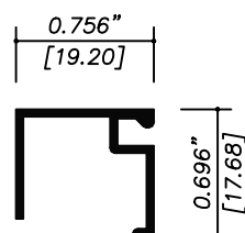
9088 JUNQUILLO
