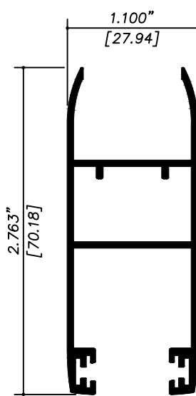
PP4010 HOJA VIDRIO DOBLE
