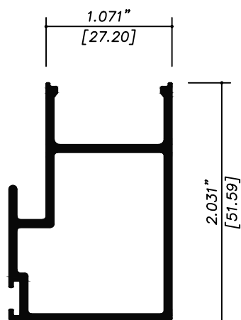
7848D TRASLAPE DUO
