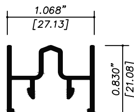
ES07 ADAPTADOR
