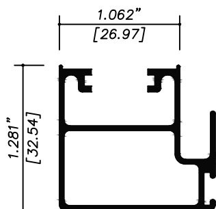
7844 TRASLAPE VENTANA
