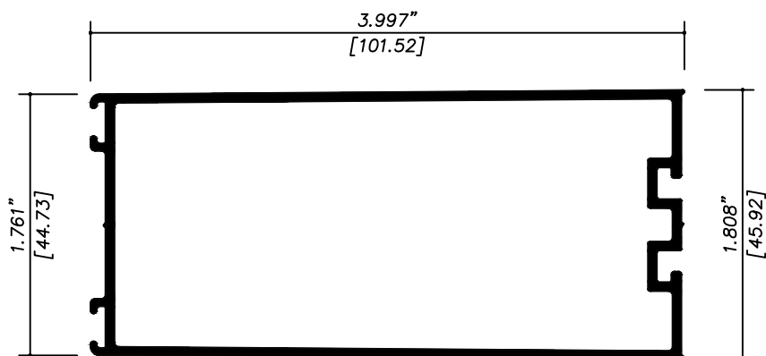
32288 CERCO RESIDENCIAL
