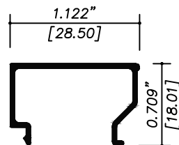
1430 JUNQUILLO ANCHO
