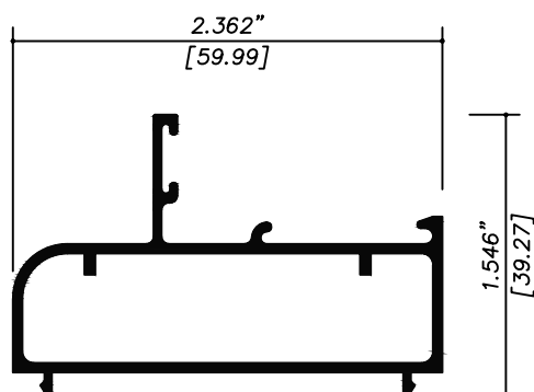
3510 FIJO TUBULAR
