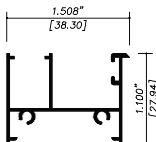
5279 JAMBA CABEZAL
