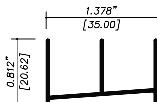
11387 RIEL VERTICAL
