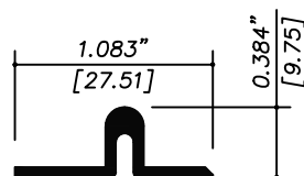
7818 ADAPTADOR 2"
