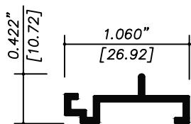
9966 ADAPTADOR MOSQUITERO
