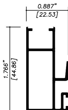
69955 TRASLAPE ESPECIAL
