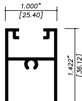
7836 CABEZAL VENTANA
