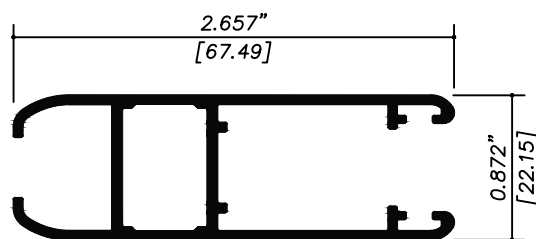
ES02 HOJA
