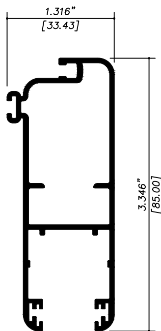
PP42198 MOSQUITERO PUERTA
