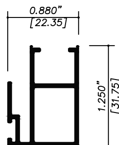
9954 TRASLAPE VENTANA
