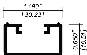
8681 CERCO FIJO 3"
