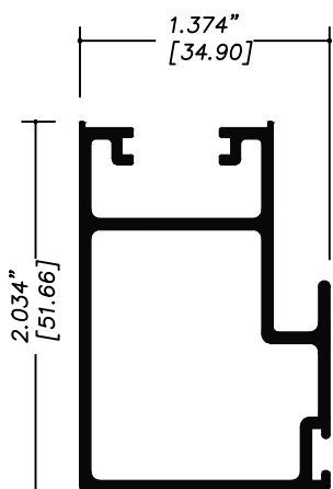
7848 TRASLAPE
