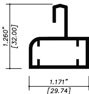
ES09 RIEL ADAPTADOR
