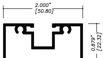
9086BC BOLSA CORTA
