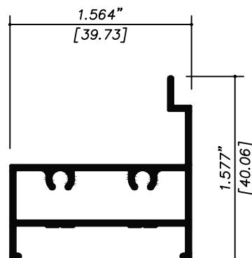
2230 CONTRA MARCO
