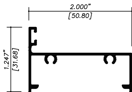
35844 BATIENTE CON VENAS ALTA
