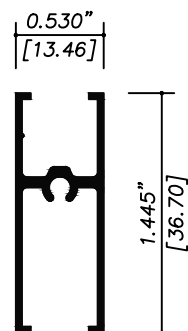
11044 CABEZAL Y ZOCLO
