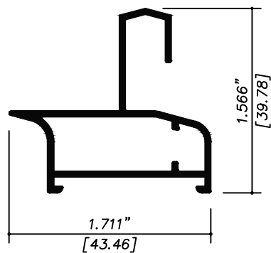
PP4006 ADAPTADOR
