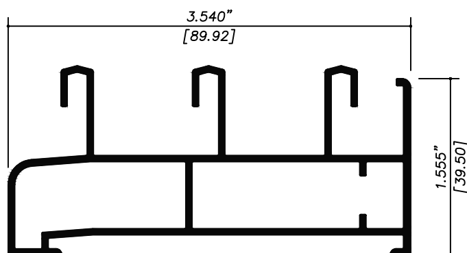
ES04 RIEL TRIPLE
