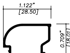
1406 HOJA LISA PUERTA
