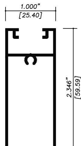
7835 ZOCLO VENTANA
