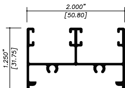
7518 CABEZAL Y JAMBA
