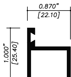
7102 BATIENTE BAÑO
