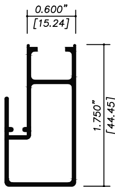
9955 TRASLAPE
