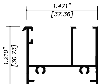
11037 JAMBA Y CABEZAL
