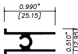
7949 MARCO
