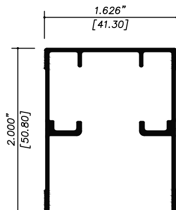
11174 RIEL SUPERIOR
