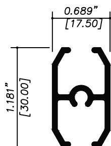
2416 CUADRICULA
