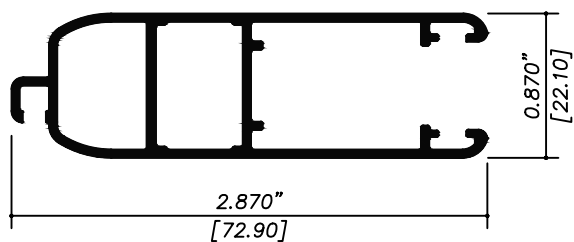
ES09 HOJA CON MOSQUITERO
