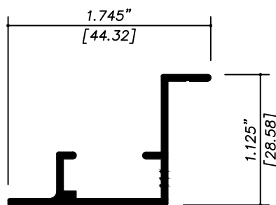
11409 RIEL SUPERIOR
