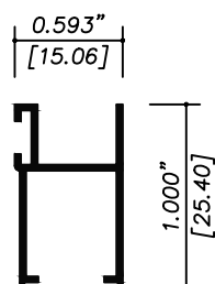
11041 CERCO TRASLAPE
