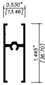
11044 CABEZAL Y ZOCLO
