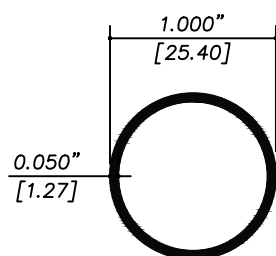
2121 REDONDO DE 1"
