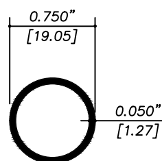
2108 REDONDO DE 3/4"
