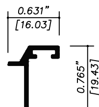
10220 ADAPTADOR OXXO
