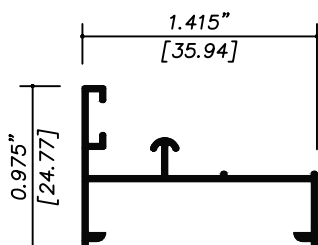
5280 RIEL
