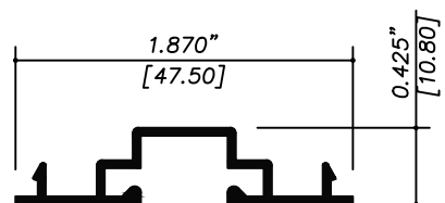
9085 TAPA BOLSA
