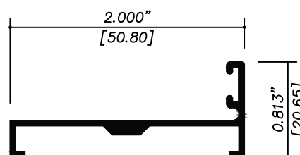
5844 BATIENTE SIN VENAS
