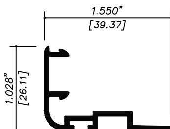
ES03 TAPA TRASLAPE
