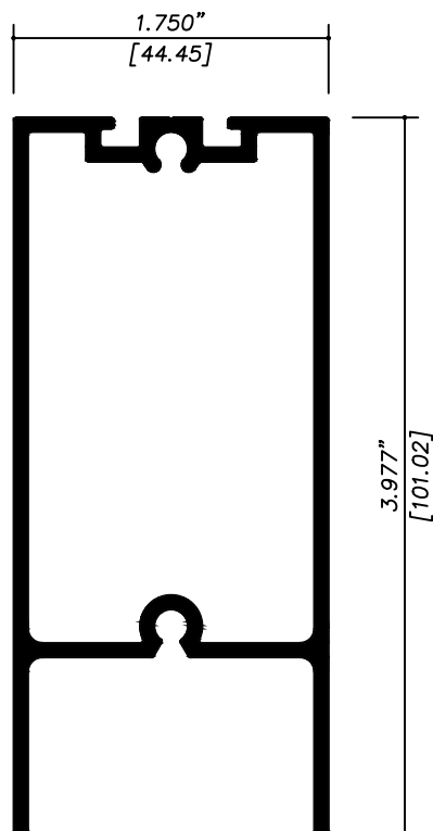
32278 ZOCLO RESIDENCIAL
