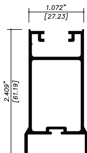
7850 CERCO OXXO
