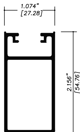
7895 CERCO CHAPA
